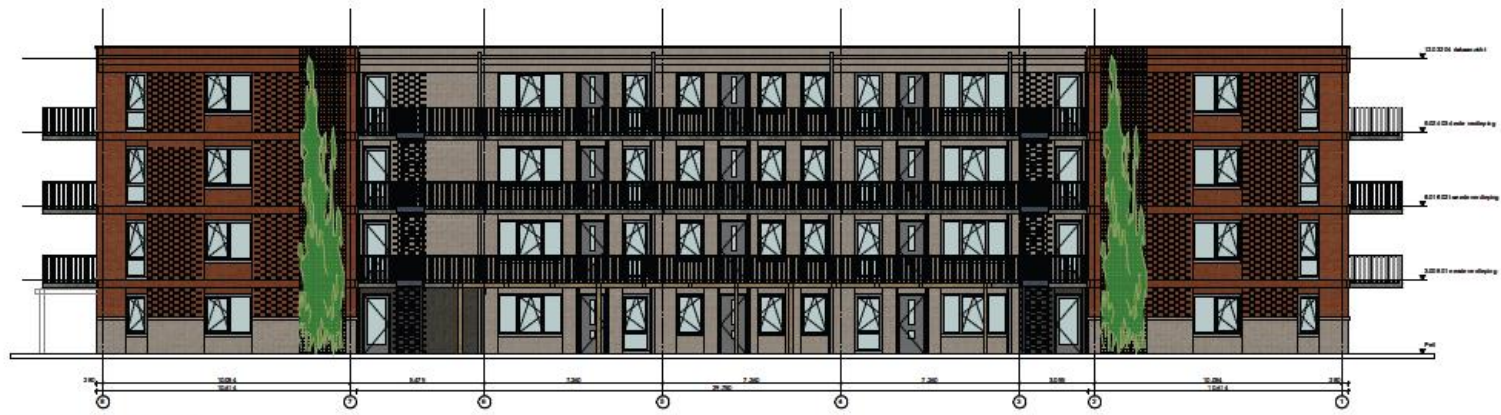
NOORDGEVEL
