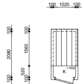
Berging1 GO wonen 0,00m 2
